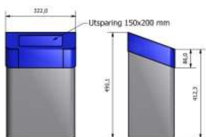
Skrå sekkeskjuler redusert innkast (art.nr: 290611)
