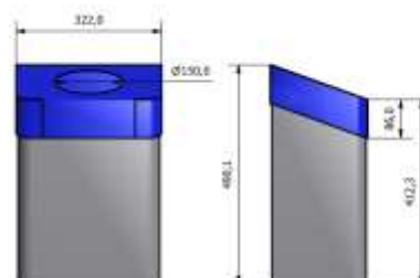
Skrå topp med utsparring flaske (art.nr: 290617) Skrå topp utskåret sirkel m/ gummileppe (art.nr: 290616)
